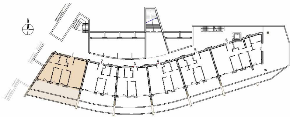
PLANIMETRIA P2
