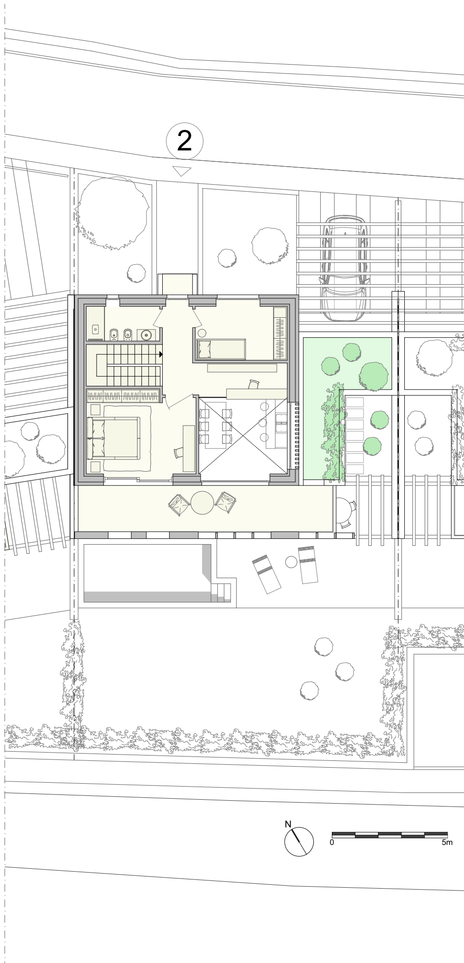
Pianta Piano Primo - Residenza n.2
