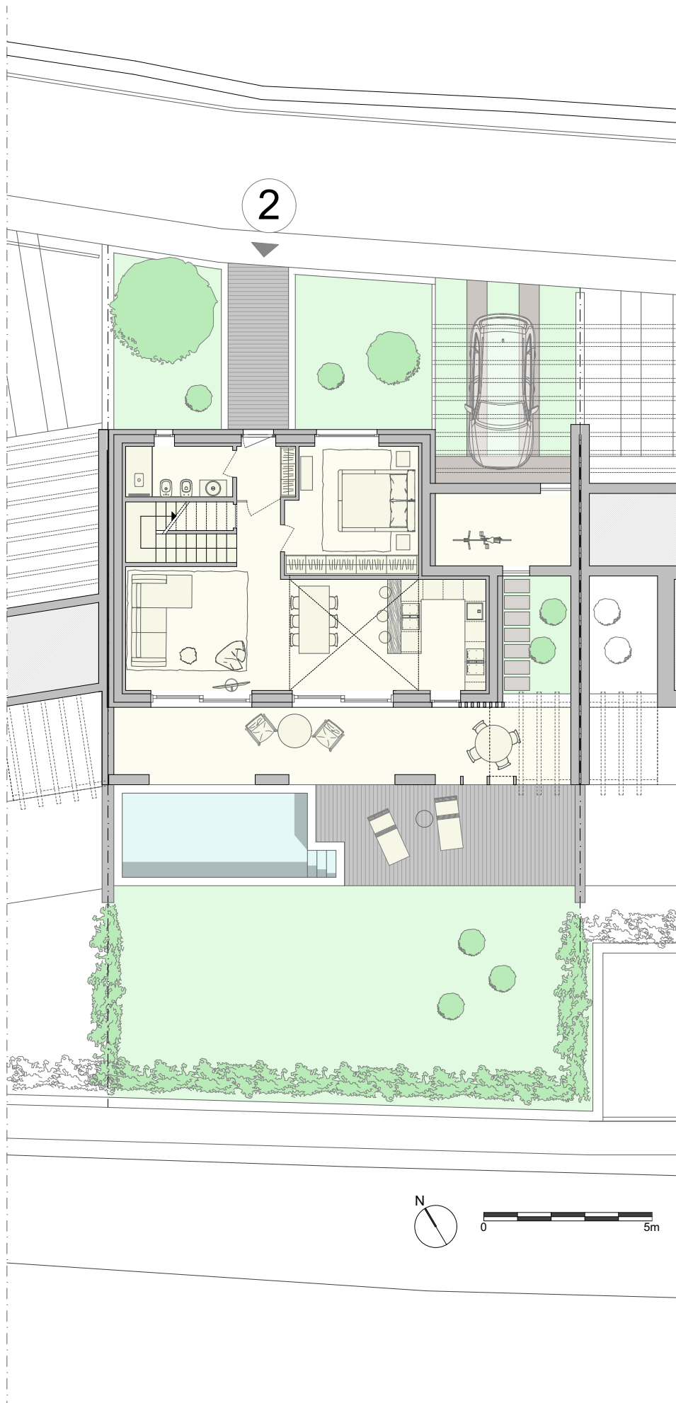
Pianta Piano Terra - Residenza n.2
