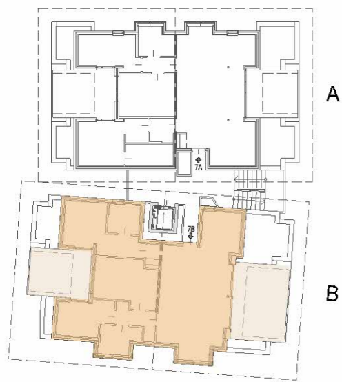
PLANIMETRIA PIANO TERZO
