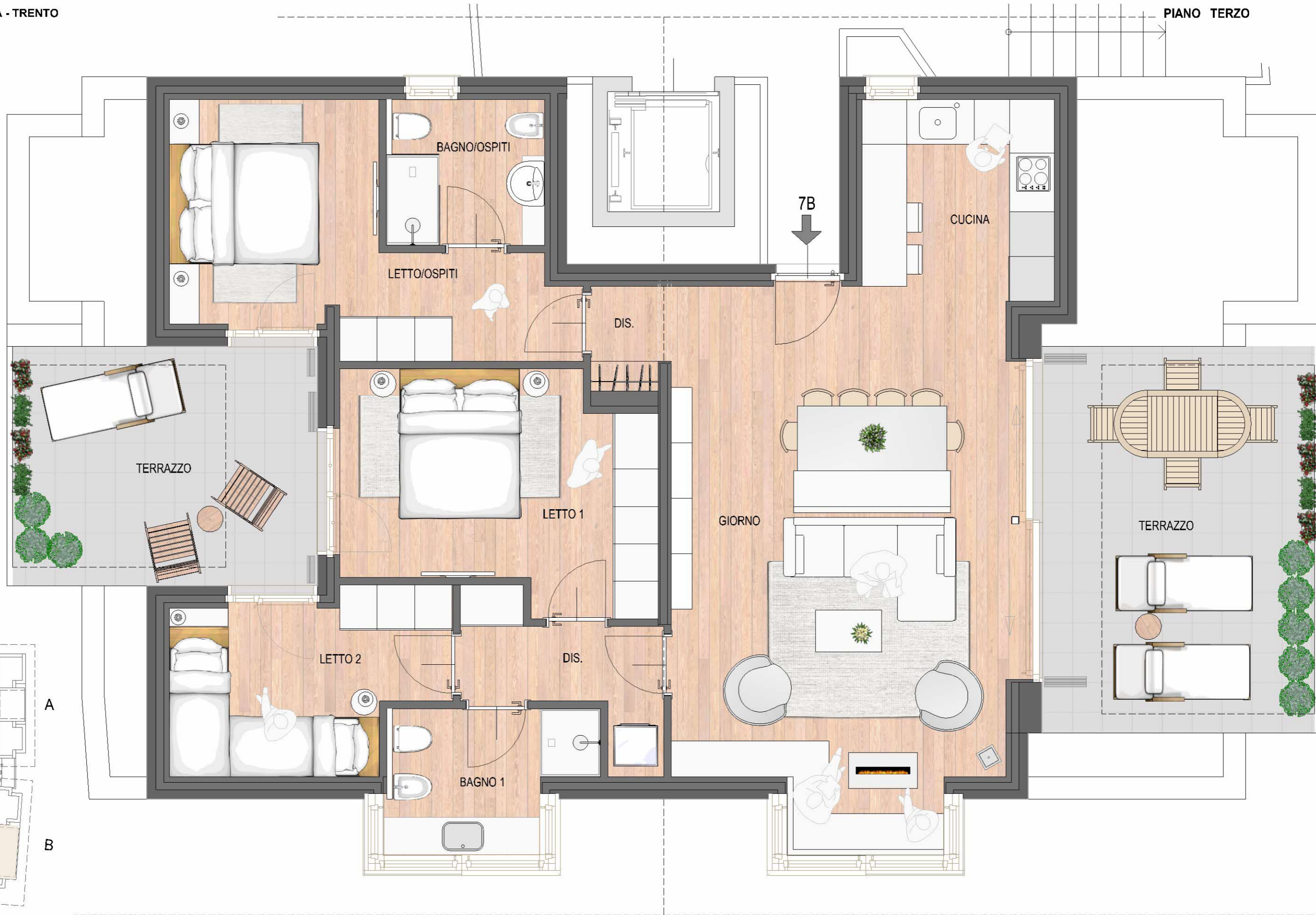
PLANIMETRIA PIANO TERZO
